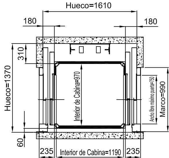
ACCESOS A 180 GRADOS
