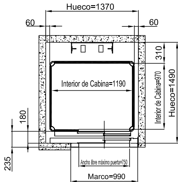
ACCESO FRONTAL PUERTA LATERAL DERECHA - IZQUIERDA
