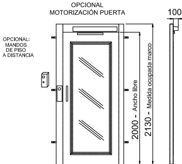
PUERTA PANORÁMICA DE CHAPA
