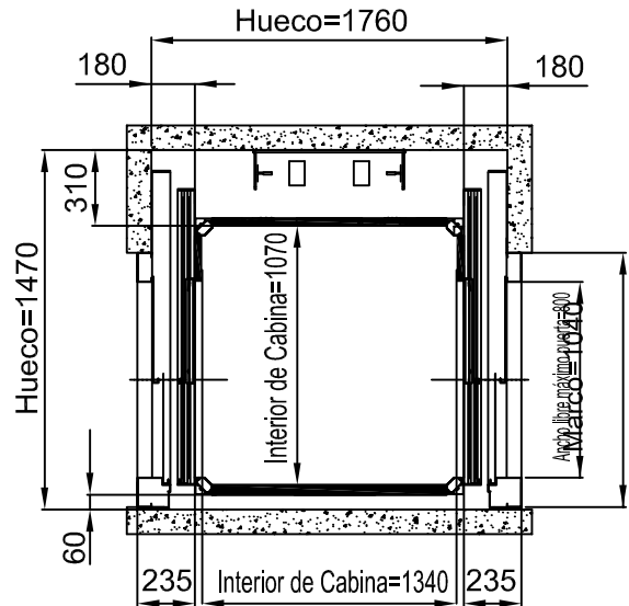
ACCESO FRONTAL PUERTA LATERAL DERECHA - IZQUIERDA
