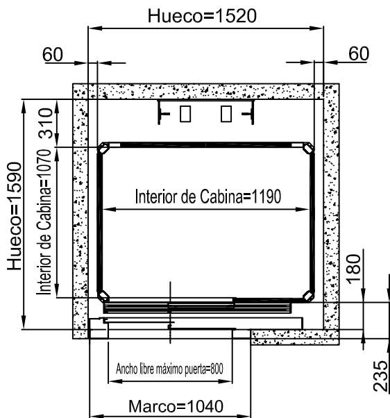
ACCESO FRONTAL PUERTA LATERAL DERECHA - IZQUIERDA
