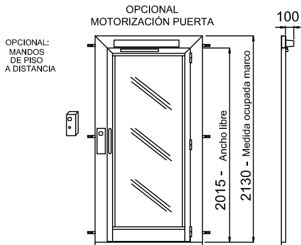
PUERTA PANORÁMICA DE ALLUMINIO
